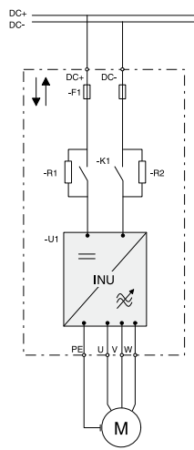
Модуль инвертора (FI9-FI14)
