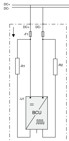
Модуль тормозного прерывателя
