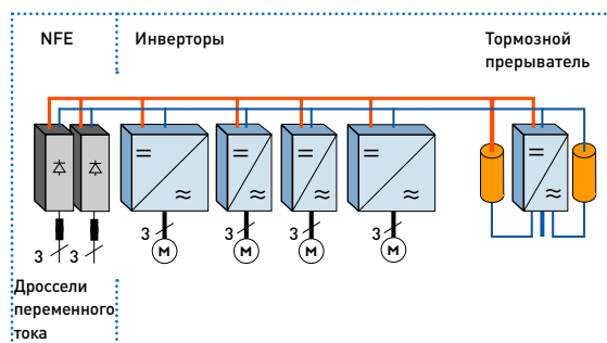
Система с общей шиной постоянного тока без функции регенерации
