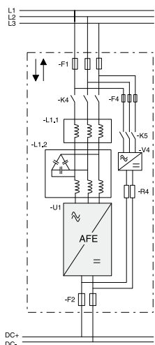
Активное входное устройство
