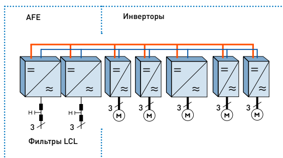
Система с общей шиной постоянного тока и с функцией регенерации
