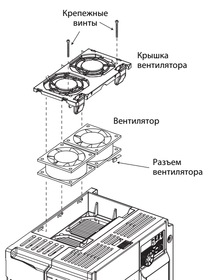
Пример FR-D740-160
