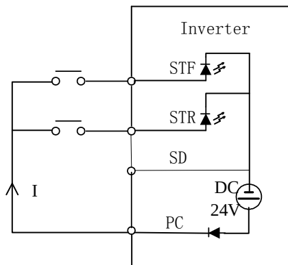
Source-режим. Дискретные входы замыкаются через «сухие контакты» непосредственно на PC
